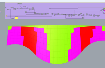
主入口雨篷龙骨模型
