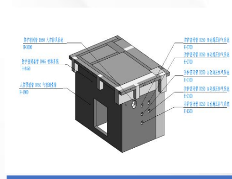
人防墙预留洞深化
