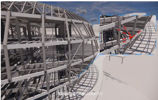
多杆件多角度汇聚概况
