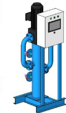
全自动胶球清洗装置-发球机
