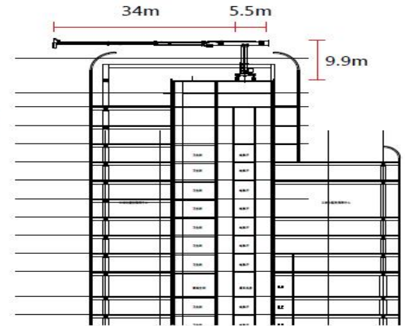
工作状态：经滑轨移动至工作位置伸缩
