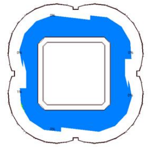
内区采光达标率分析彩图(31F)
