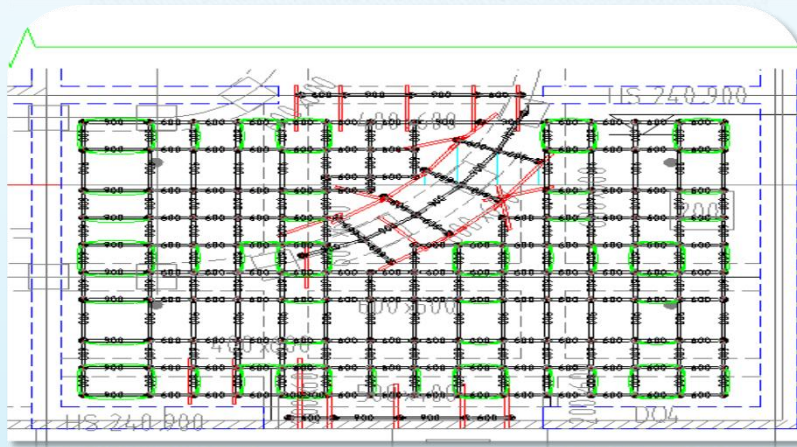
BIM模板架体支撑出图
