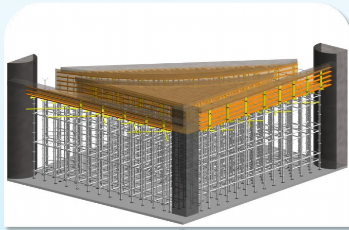
BIM模板架体支撑深化模型
