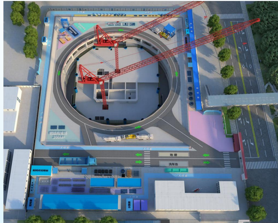
现场塔吊设置
