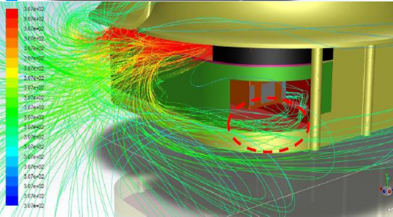
冷却塔方案一出风轨迹图
