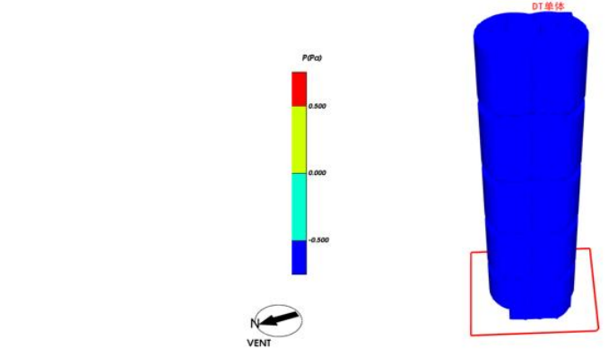
建筑背风面外窗表面风压云图-夏季/过渡季
